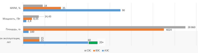
Выработка электроэнергии АЭС и ВИЭ с учетом показателя КИУМ
